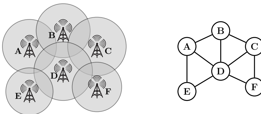
FIGURE 1 – Modélisation d’un réseau d’antennes par un graphe d’interférence.
